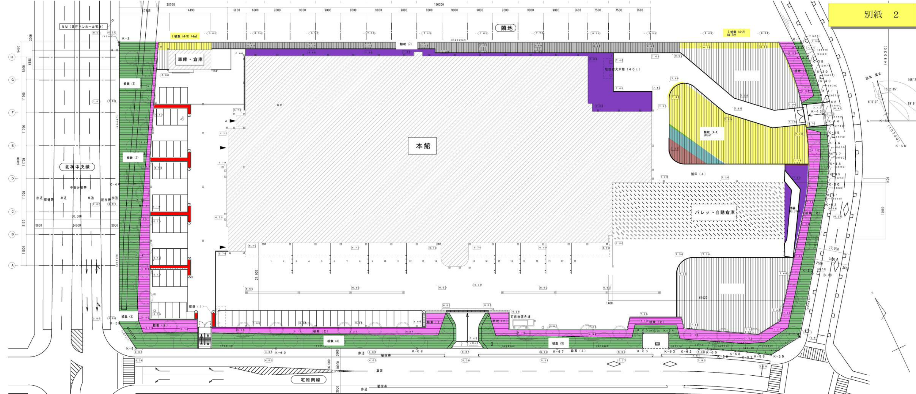
外構植栽平面図 1/400
